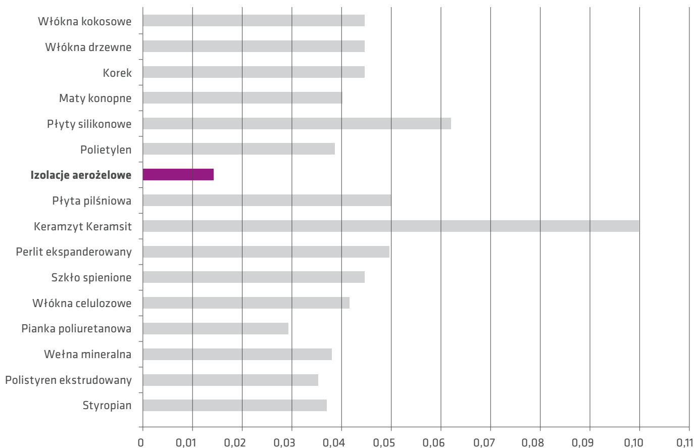
WSPÓŁCZYNNIK PRZEWODZENIA CIEPŁA λ [W/(mK)]
