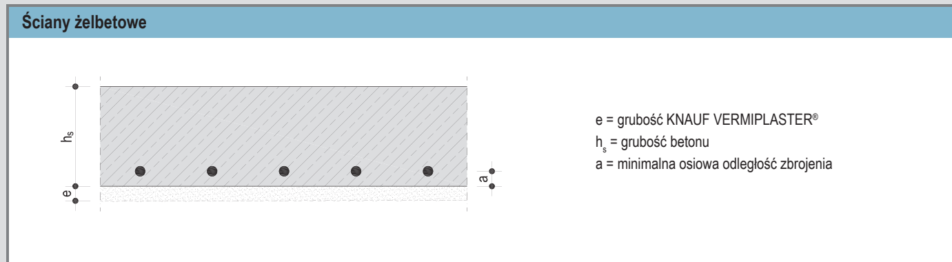
Wartości odpowiadającej grubości betonu wg Europejskiej Aprobaty Technicznej ETA-11/0229
