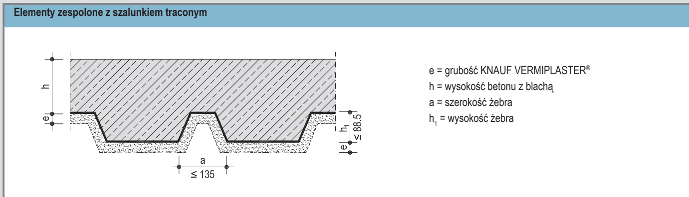
Minimalna grubość naniesionego tynku gipsowego Knauf VERMIPLASTER®
